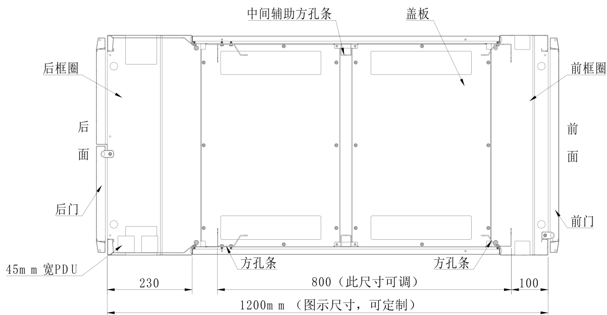
图 17: 机柜内部方孔条安装位置示意图
