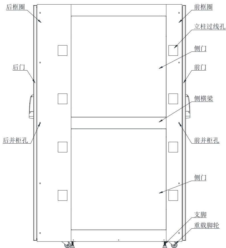
图 26: 机柜侧面示意图
